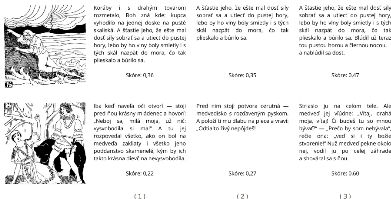
Obr. 5 Porovnanie úspešnosti sémantického párovania textových úryvkov k ilustráciám z rozprávky Trojruža pri použití modelov (1) S-BERT (MiniLM) , (2) anglický S-BERT (all-mpnet-base-v2) a (3) SlovakBERT .
