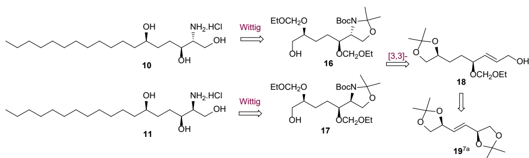
Obr. 7 Retrosyntetická stratégia vedúca k cieľovým sfingoidným bázam 10 a 11 .
