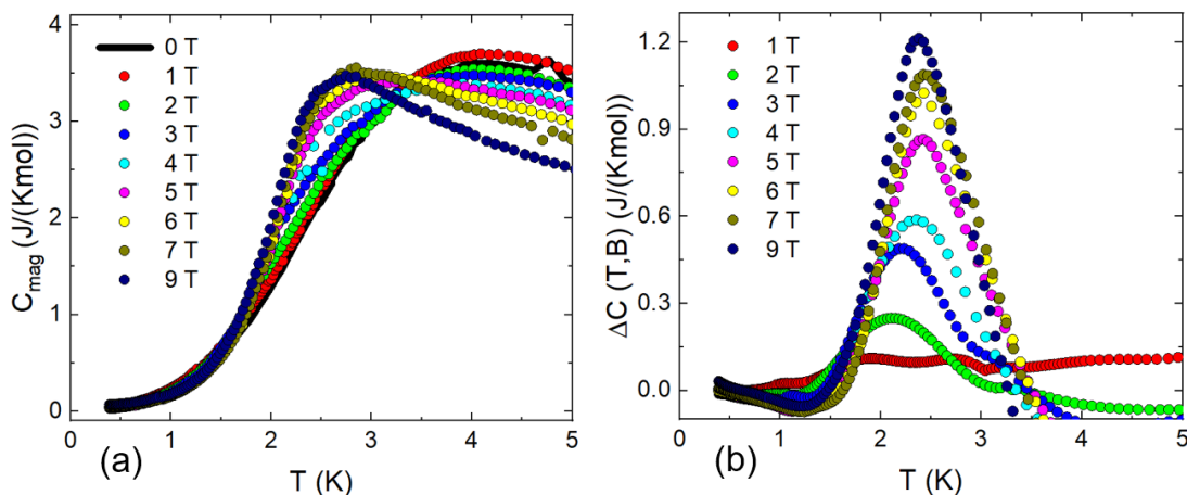
Obr. 5. (a) Teplotné závislosti magnetického príspevku tepelnej kapacity C_{mag} v magnetických poliach až do 9 T. (b) Rozdiely \Delta C(T, B) magnetického príspevku tepelnej kapacity meranou v aplikovanom C(T, B) a v nulovom poli C(T, 0) pre jednotlivé hodnoty vonkajších polí B .
