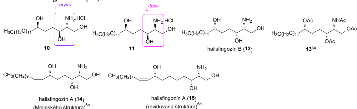
Obr. 6 Štruktúra našich cieľových molekúl 10, 11 a porovnanie s halisfingozínom B (12). Predpokladaná a revidovaná štruktúra halisfingozínu A.
