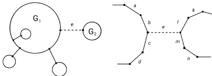
Obr. 3 Rovinný graf s mostami
