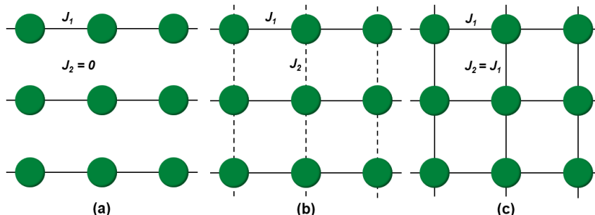
Obr. 2. Schematické znázornenie rôznych variantov anizotropie výmennnej interakcie v prípade dvojrozmernej mriežky: (a) R = 0 , (b) 0 < R < 1 , a (c) R = 1 .
