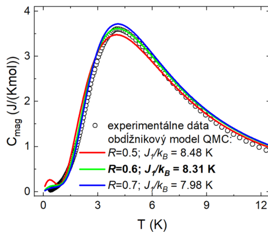
Obr. 4. Teplotná závislosť magnetického príspevku tepelnej kapacity a jej porovnanie s výsledkami QMC výpočtov pre vybrané hodnoty parametra anizotropie R (a im zodpovedajúce hodnoty dominantnej výmennej interakcie J_I/k_B ).
