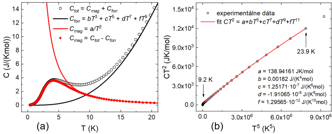
Obr. 2. (a) Teplotné závislosti magnetického príspevku C_{mag} , fonónového príspevku C_{fon} a celkovej tepelnej kapacity C_{tot} pre \text{Cu}(\text{pm})(\text{ea})_2 v nulovom magnetickom poli. (b) Fit experimentálnych dát celkovej tepelnej kapacity podľa vzťahu (2) v teplotnom intervale 9.2 K až 23.9 K.
