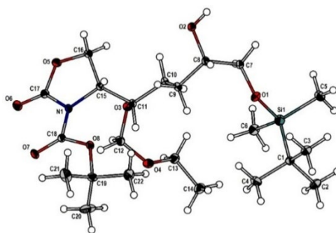
Obr. 8 ORTEP štruktúra oxazolidinónu 32 s príslušným kryštalografickým číslovaním.
