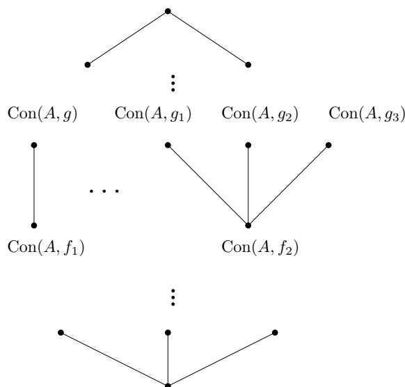
Obr. 1: Príklad zväzu \mathcal{E}_A
