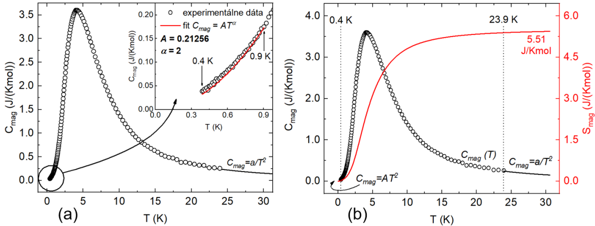
Obr. 3. (a) Teplotná závislosť magnetického príspevku tepelnej kapacity C_{mag}(T) (body) a jej interpolácia do vyšších teplôt C_{mag} = a/T^2 (plná čiara). Vnútro zobrazuje fit nízko-teplotného intervalu. (b) Teplotná závislosť C_{mag} (ľavá os) a magnetickej zložky entropie S_{mag} (pravá os).
