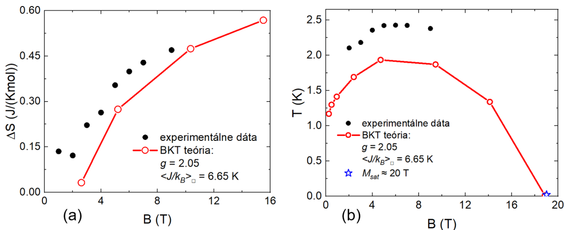
Obr. 6. (a) Poľná závislosť entropie \Delta S(T, B) v magnetickom poli pre jednotlivé hodnoty vonkajšieho poľa a jej porovnanie s teóriou pre poľom indukovaný BKT prechod pre S = 1/2 2D Heisenbergov antiiferomagnet na izotropnej štvorcovej mriežke s \langle J/k_B \rangle_{\square} = 6.65 \text{ K} . (b) Magnetický fázový diagram a jeho porovnanie s teóriou pre poľom indukovaný BKT prechod pre S = 1/2 2D Heisenbergov antiiferomagnet na izotropnej štvorcovej mriežke s \langle J/k_B \rangle_{\square} = 6.65 \text{ K} .
